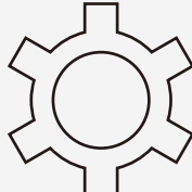
制造业
